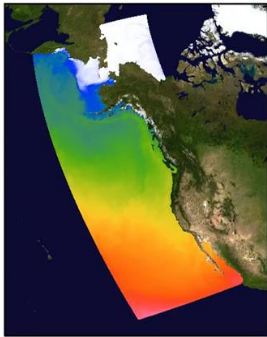
1980-04-16 sea surface temperature (°C) 0 5 10 15 20 25 30
