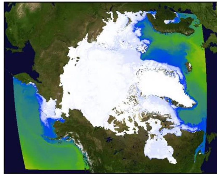
1980-04-16 sea surface temperature (°C) 0 5 10 15 20 25 30
